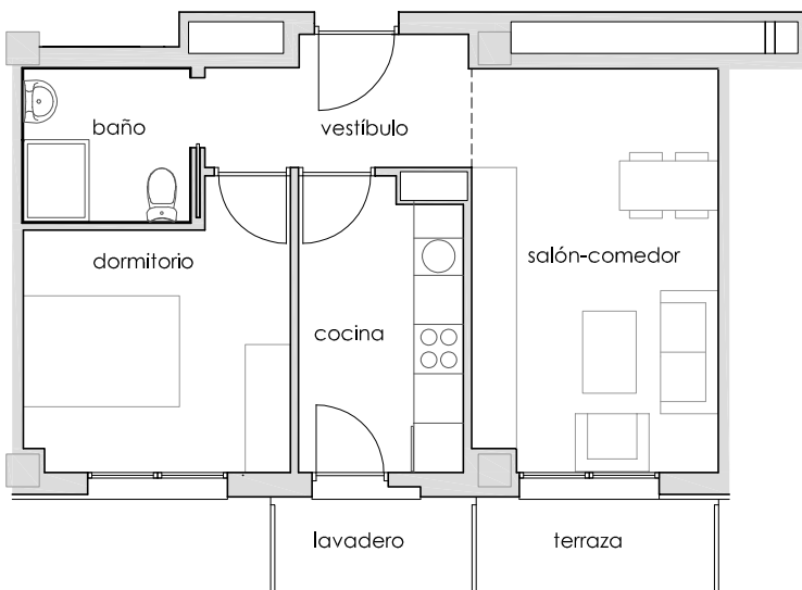
Situación vivienda 1ºB. Planta primera. E: 1/300
