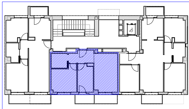
Situación vivienda 1ºB. Planta primera. E: 1/300
