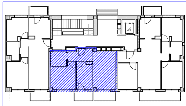
Situación vivienda 3ºB. Planta tercera. E: 1/300
