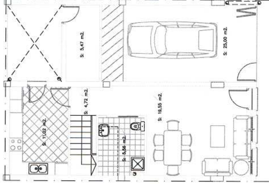
PLANTA BAJA
