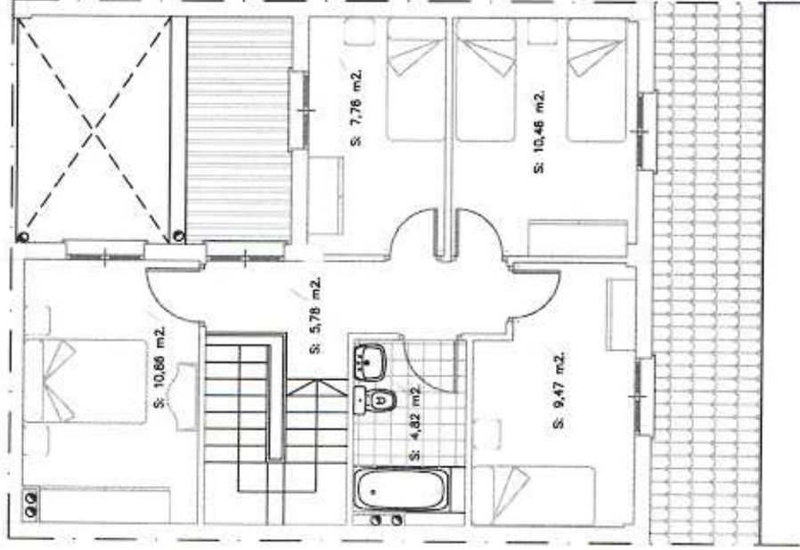
PLANTA PRIMERA
